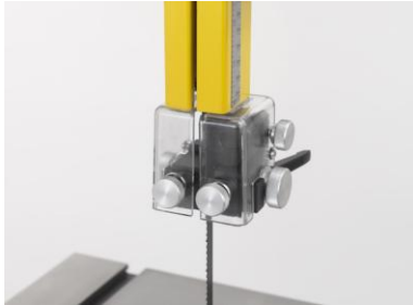
Werkzeuglos einstellbare Gleitblock-Sägeföhrungen
